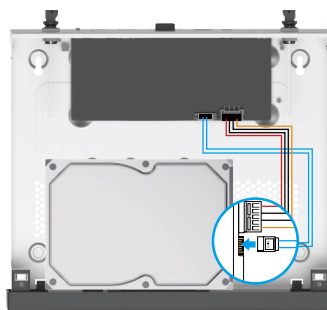
Ligação do cabo de dados
