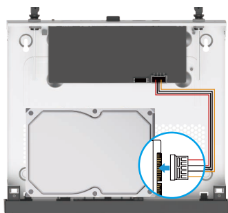
Ligação do cabo de alimentação
